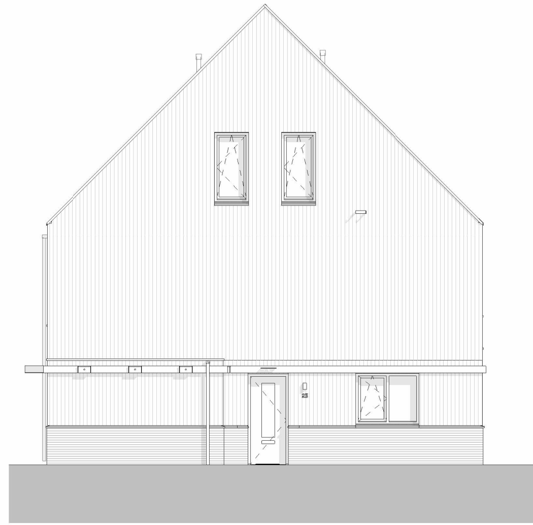
zijgevel (oost)
