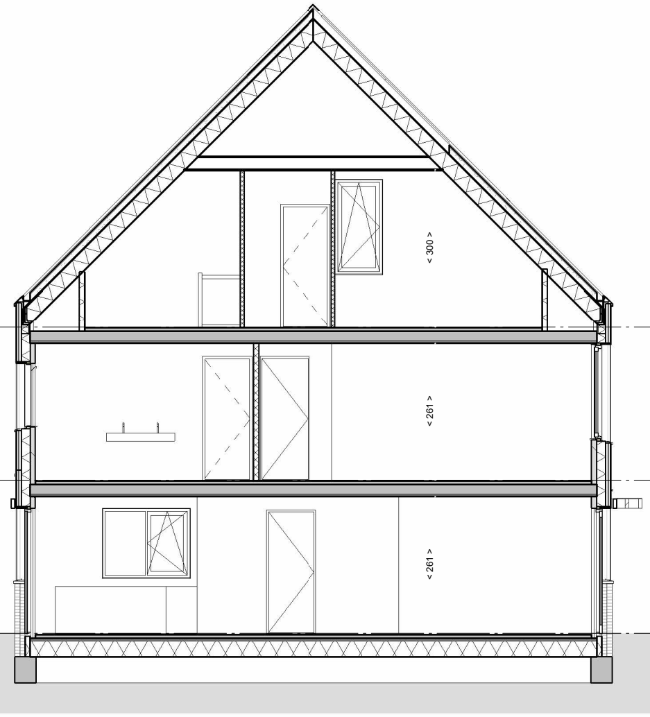
dwarsdoorsnede
