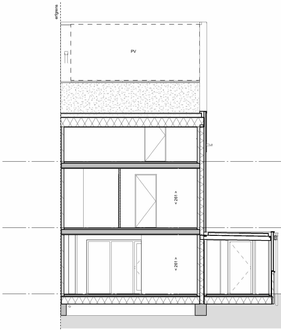
langsdoorsnede
